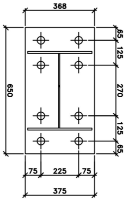
BASE PLATE D1
