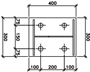
BASE PLATE D2
