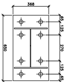
BASE PLATE D2A & D2B
